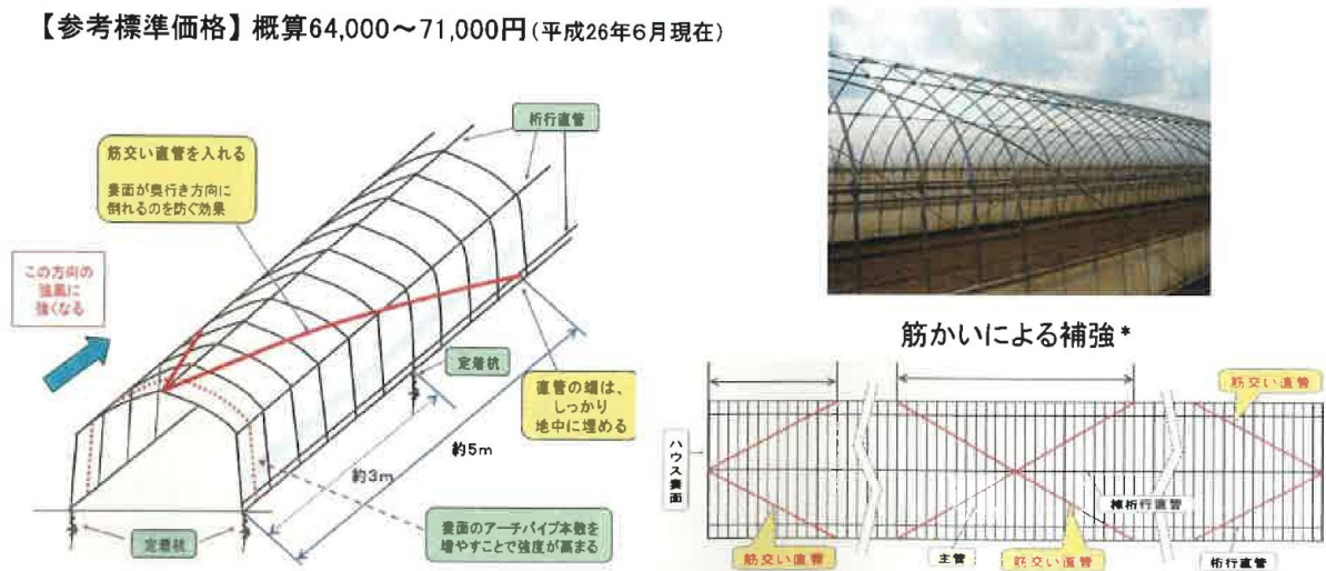
筋かいによる妻面の補強方法事例
