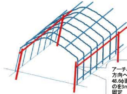
側面補強の参考例
